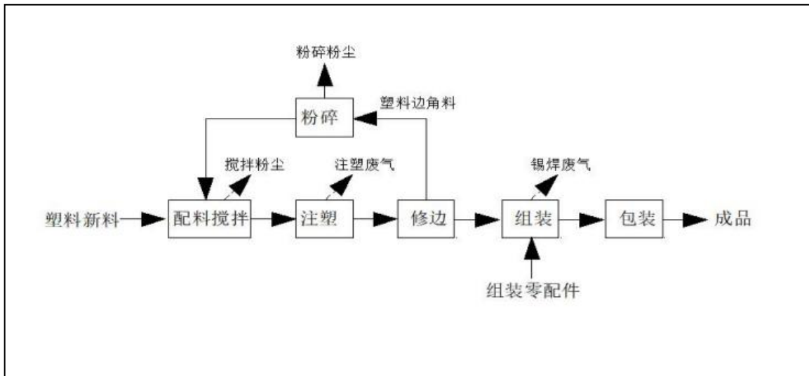
图 2-3 生产工艺流程图
