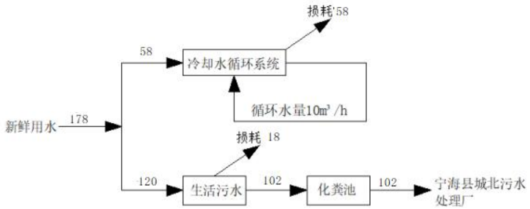
图 2-4 水平衡图 单位：t/a
